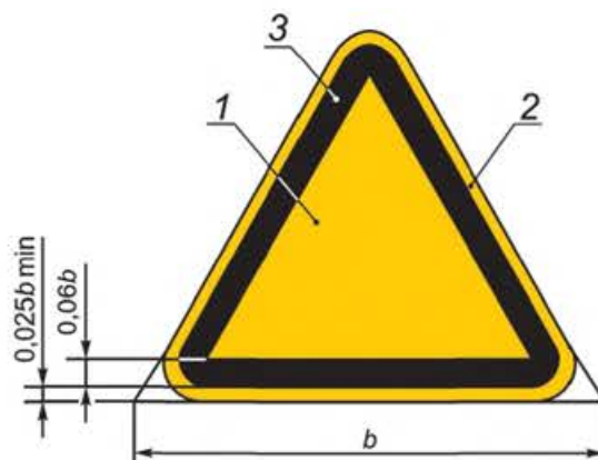
b — сторона треугольника; 1 — основная поверхность; 2 — кант; 3 — кайма
