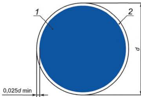
d — диаметр круга; 1 — основная поверхность; 2 — кант
